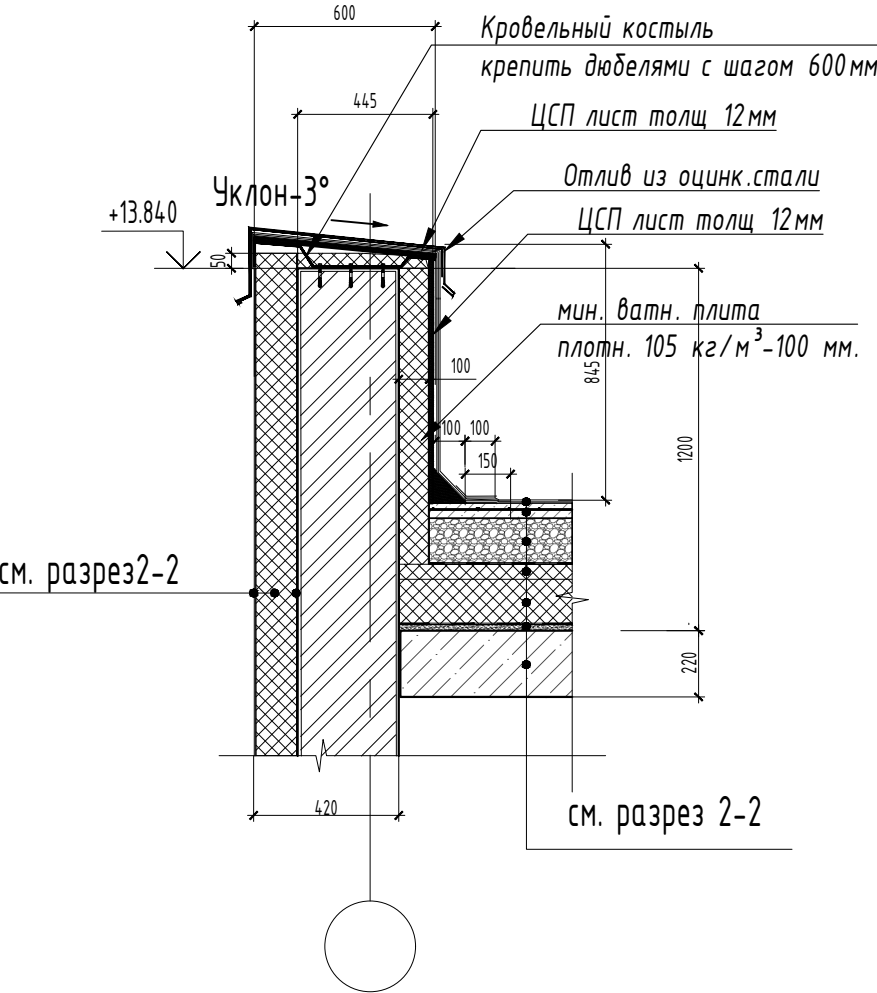
Парапет кирпичный.
