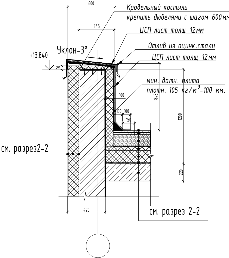
Парапет кирпичный.
